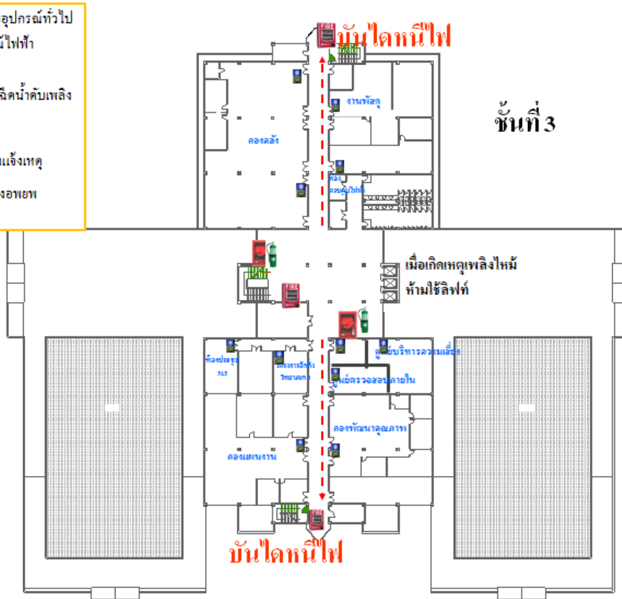
แผนผังเส้นทางหนีไฟและอุปกรณ์ดับเพลิง
