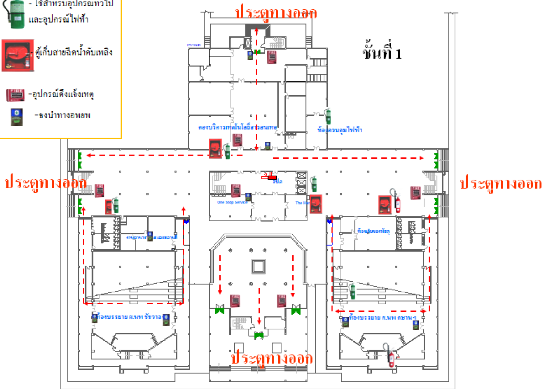
แผนผังเส้นทางหนีไฟและอุปกรณ์ดับเพลิง
